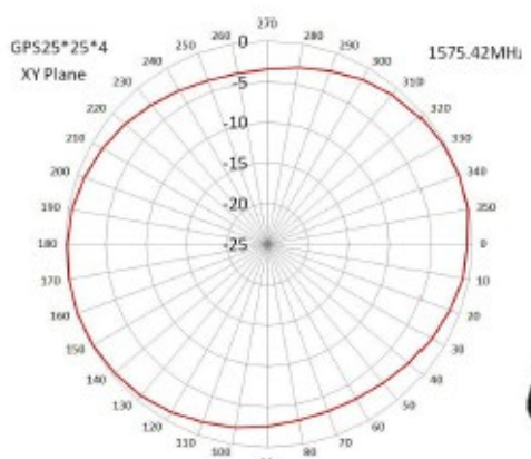
GPS Antenna
